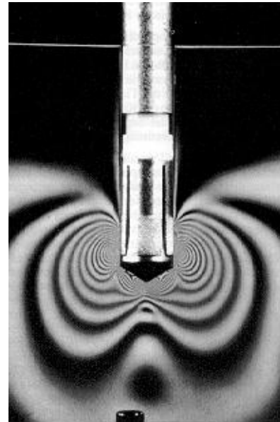
Die Spannungsverteilung der Spreizkräfte am richtig montierten Stahlanker
